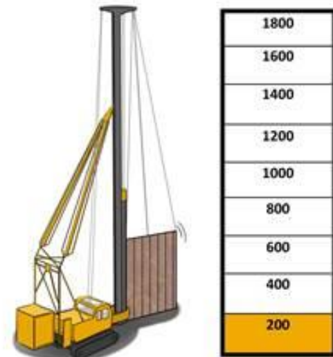
Damwanden aanbrengen
