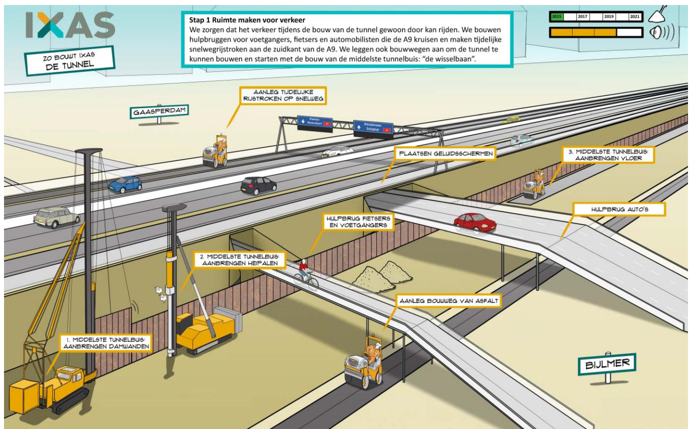
Afbeelding: IXAS maakt op dit moment ruimte voor het snelwegverkeer tijdens de bouw van de tunnel. Onderdeel daarvan is de aanleg van de wisselbaan. De heipalen zijn daar weer een onderdeel van.
